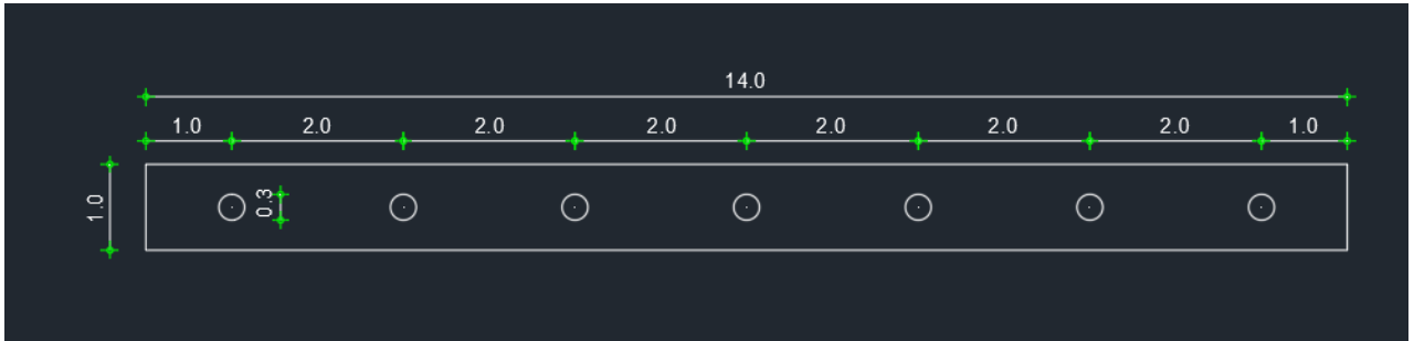
Σχέδιο Διάτρησης
