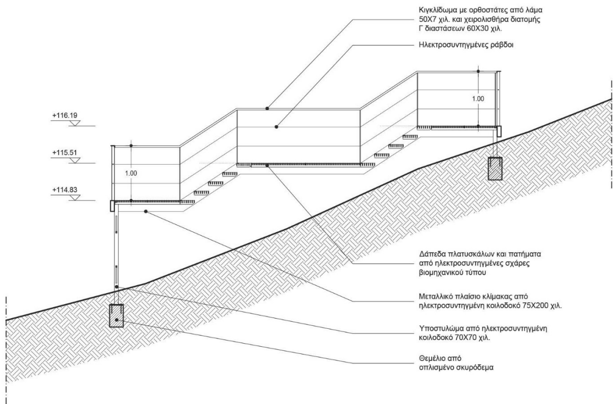
Τομή A-A
