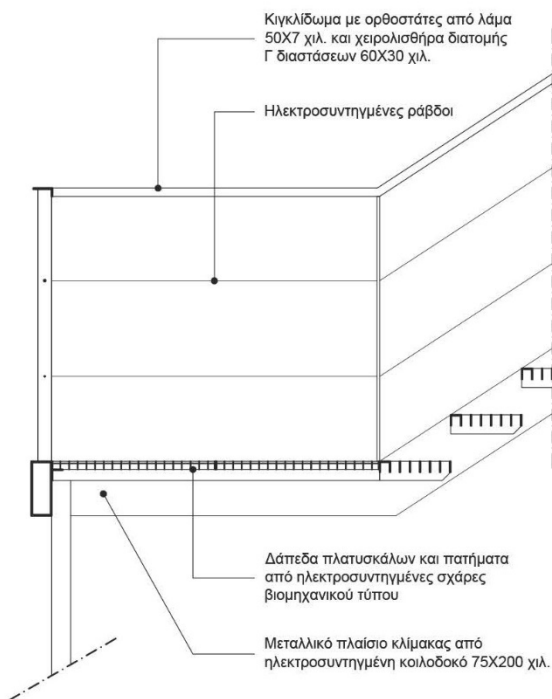
Λεπτομέρεια Κατασκευαστική
